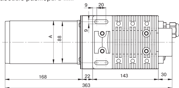
Базовые размеры в мм
