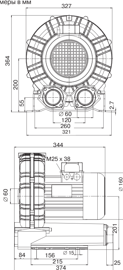
Базовые размеры в мм
